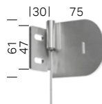
Universalträger mit Seilführung
